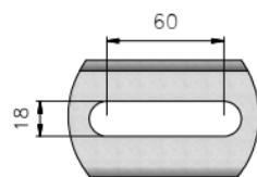
DETALHE 2 RASGO OBLONGO PEÇA 2
