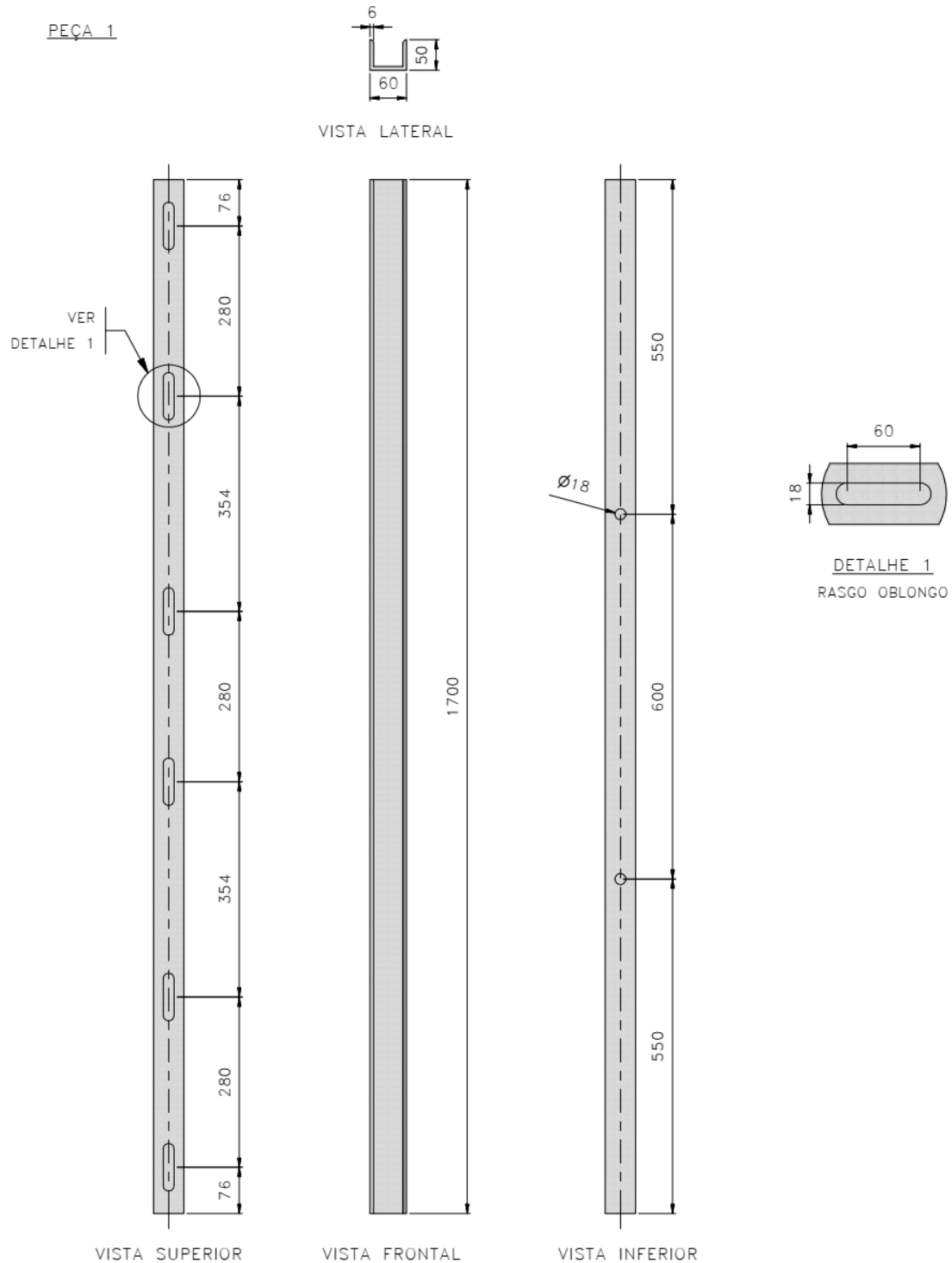
Figura 1 - Detalhes da peça 1
