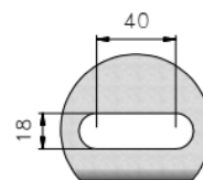
DETALHE 3 RASGO OBLONGO PEÇA 3
