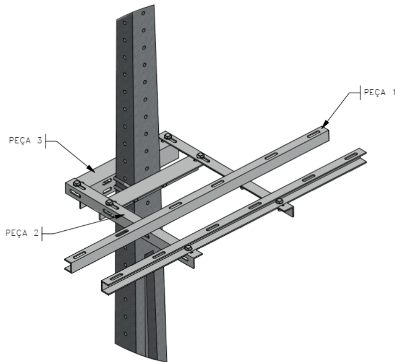
VISTA EM PERSPECTIVA CONJUNTO MONTADO EM POSTE
